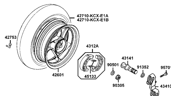
F8 後輪 Rear Wheel
