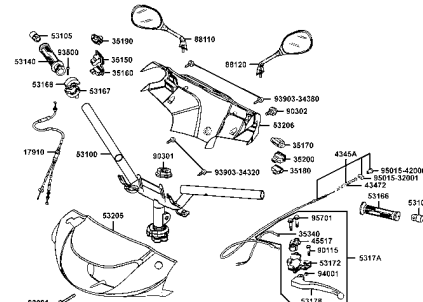
F6 轉向桿●前避震器 Front Cushion
