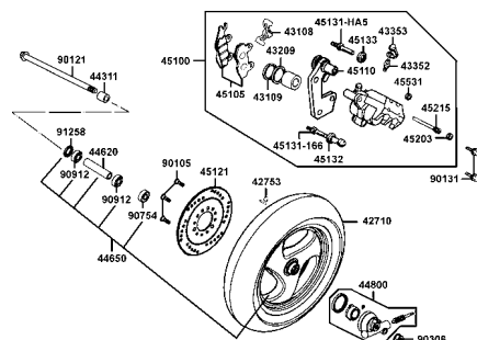
F7 前輪 Front Wheel
