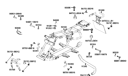
F18 Frame Body
