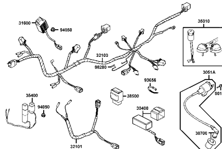
F17 Wire Harness
